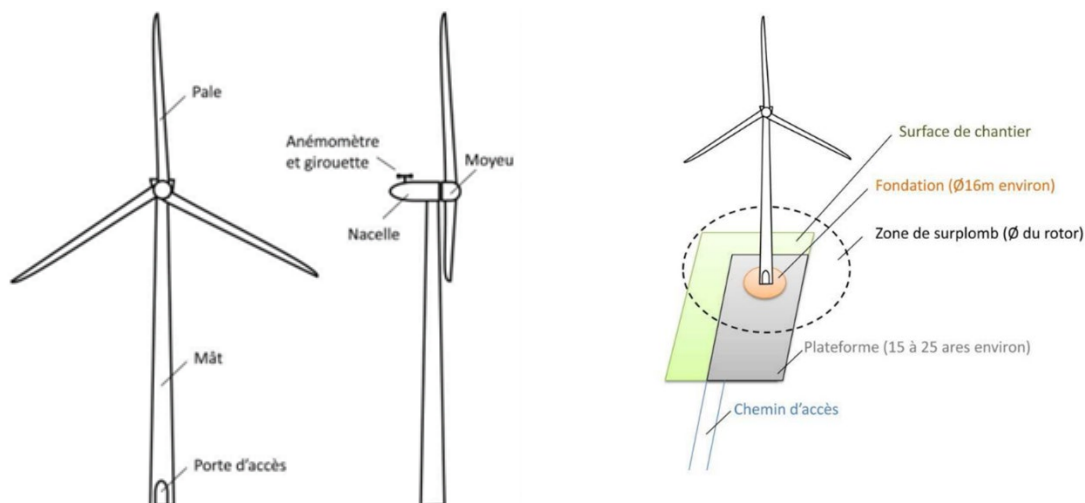
Représentation schématique d'une éolienne (source : SOLVEO Energies)
